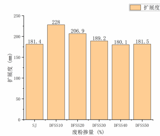
图 7 砂浆扩展度随掺量的变化情况 Fig. 7 Variation of the mortar flow spread diameter
