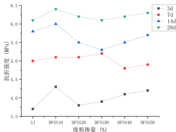
图 8 DFSS 系列抗折强度变化情况
