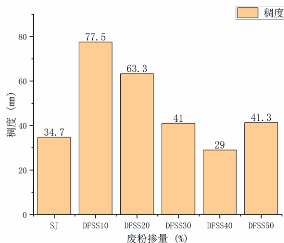
图 6 砂浆稠度随废粉掺量的变化情况
