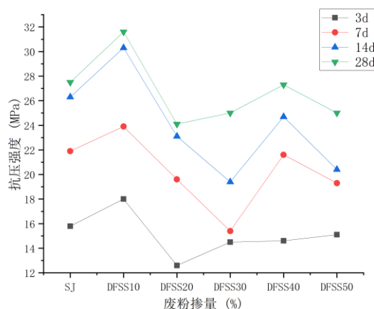
图 9 DFSS 系列抗压强度变化情况
