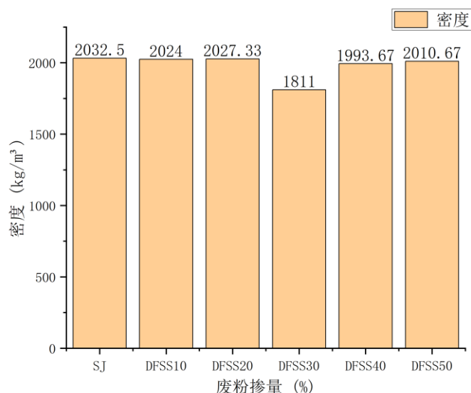
图 5 砂浆密度随掺量的变化情况
