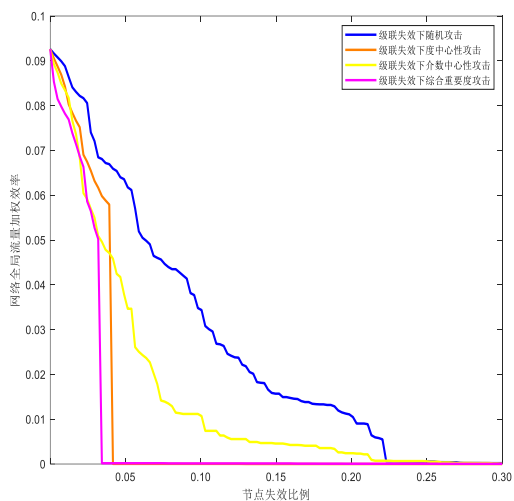
(a) \alpha=0.4 时网络全局流量加权效率变化图
