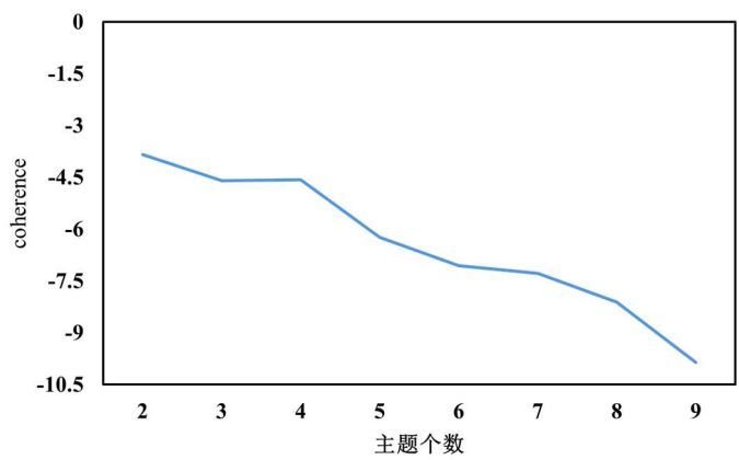
图 5 主题一致性分析结果 Fig. 5 Results of thematic coherence analysis
